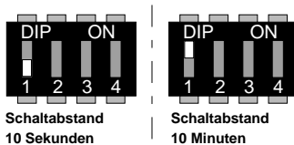
DIP-Schalter
