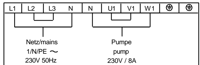
Anschluss einer 230V Wechselstrompumpe
