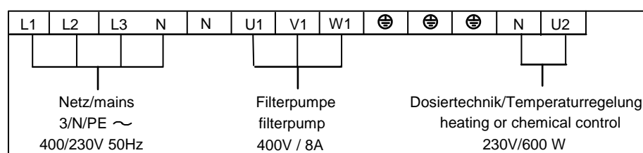
Anschluss einer 400V Drehstrompumpe
