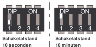
DIP-Schakelaar
